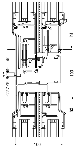
6 インペイ外倒し排煙 / 引違い
