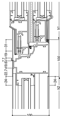
35 外動片引き / FIX
