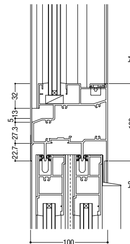
11 外動片引き / 外動片引き
