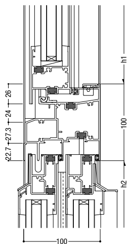
7 外倒し排煙 / 両袖可動
