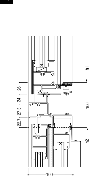
17 FIX／外動片引き
