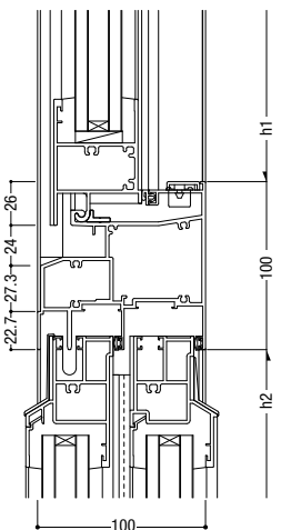
10 外動片引き / 外動片引き
