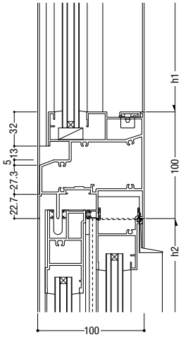
20 両袖可動 / 両袖可動
