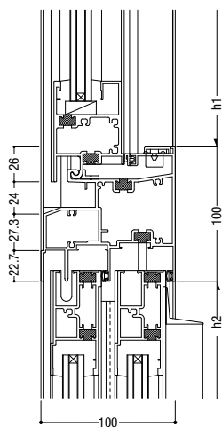
5 外倒し排煙 / 外動片引き
