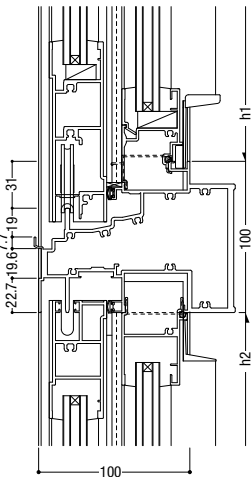
23 インペイ外倒し排煙 / 両袖可動
