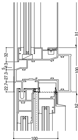
29 外開き / 外開き たてすべり出し / たてすべり出し
