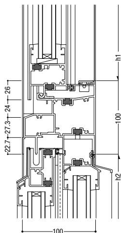
9 外倒し排煙 / 両袖可動
