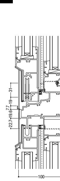
24 インペイ外倒し排煙／両袖可動
