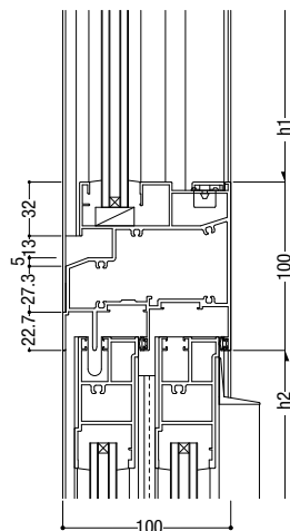
11 外動片引き / 外動片引き
