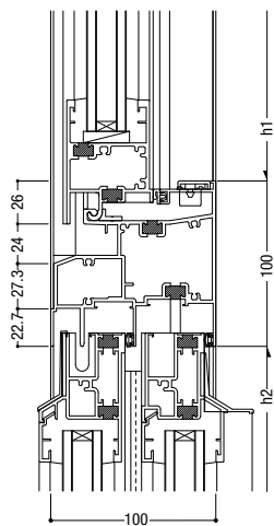
6 外倒し排煙 / 外動片引き
