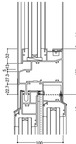
22 インペイ外倒し排煙 / 両袖可動
